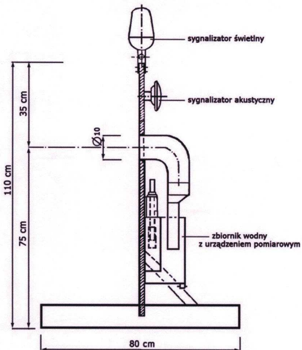
Rys. 6. Tarcza nalewowa
